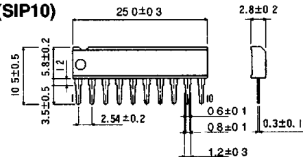
BA6886N (SIP10)
