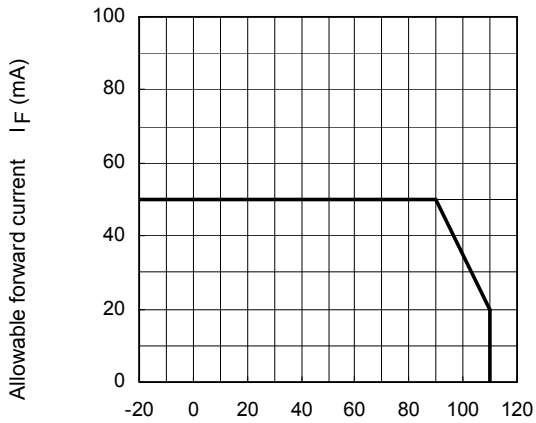
I_F - T_a
