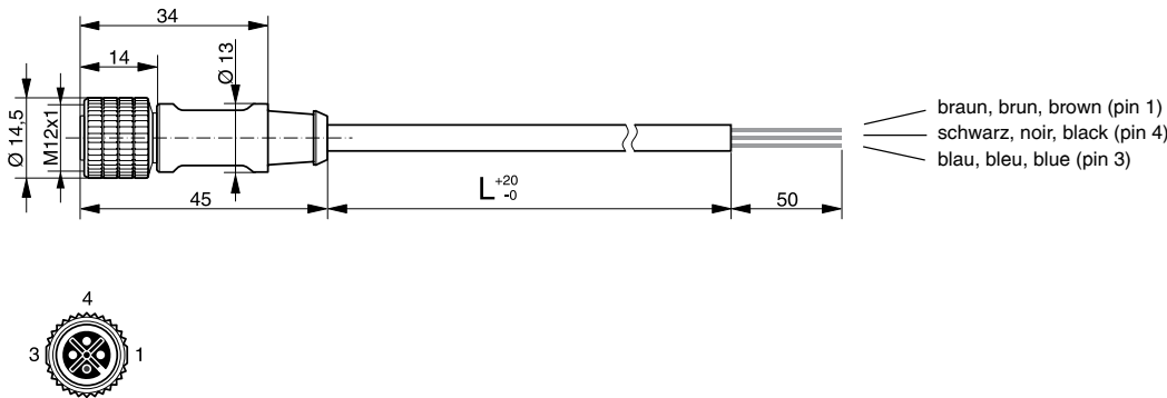
gerade / droit / straight
