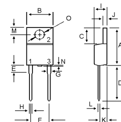
TO-220A
