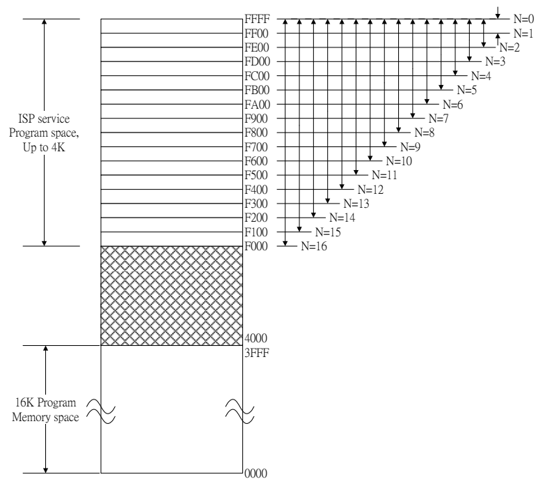
Fig. 3-3 : SM59R05G6 programmable Flash
