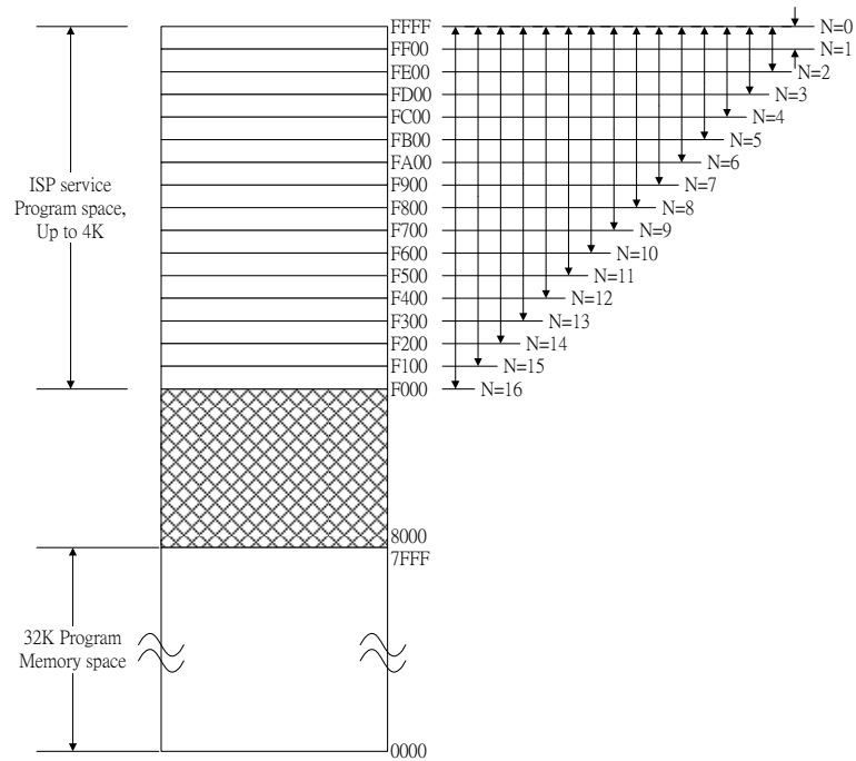
Fig. 3-2 : SM59R09G6 programmable Flash
