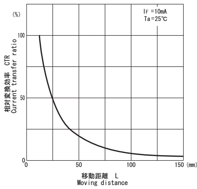
■相对変換効率/距離特性 CTR/L
