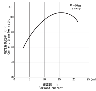
■相对変換効率/順電流特性 CTR/I_f
