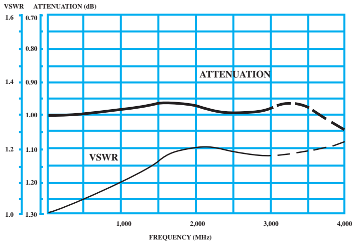
1 dB ATTENUATOR
