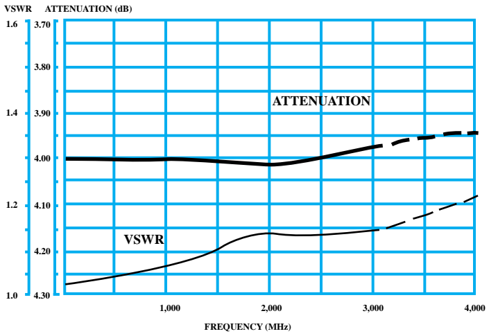
4 dB ATTENUATOR
