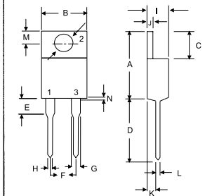
TO-220A
