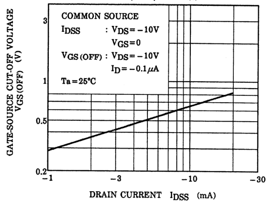
V_{GS(OFF)} - I_{DSS}
