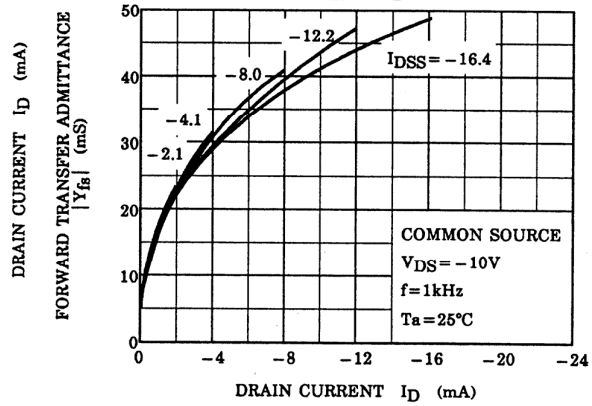
|Y_{fs}| - I_D
