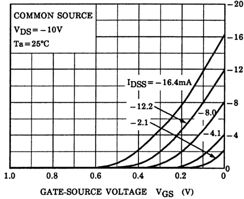
I_D - V_{GS}
