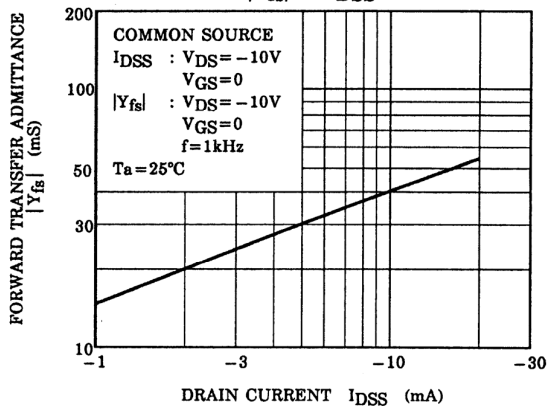
|Y_{fs}| - I_{DSS}
