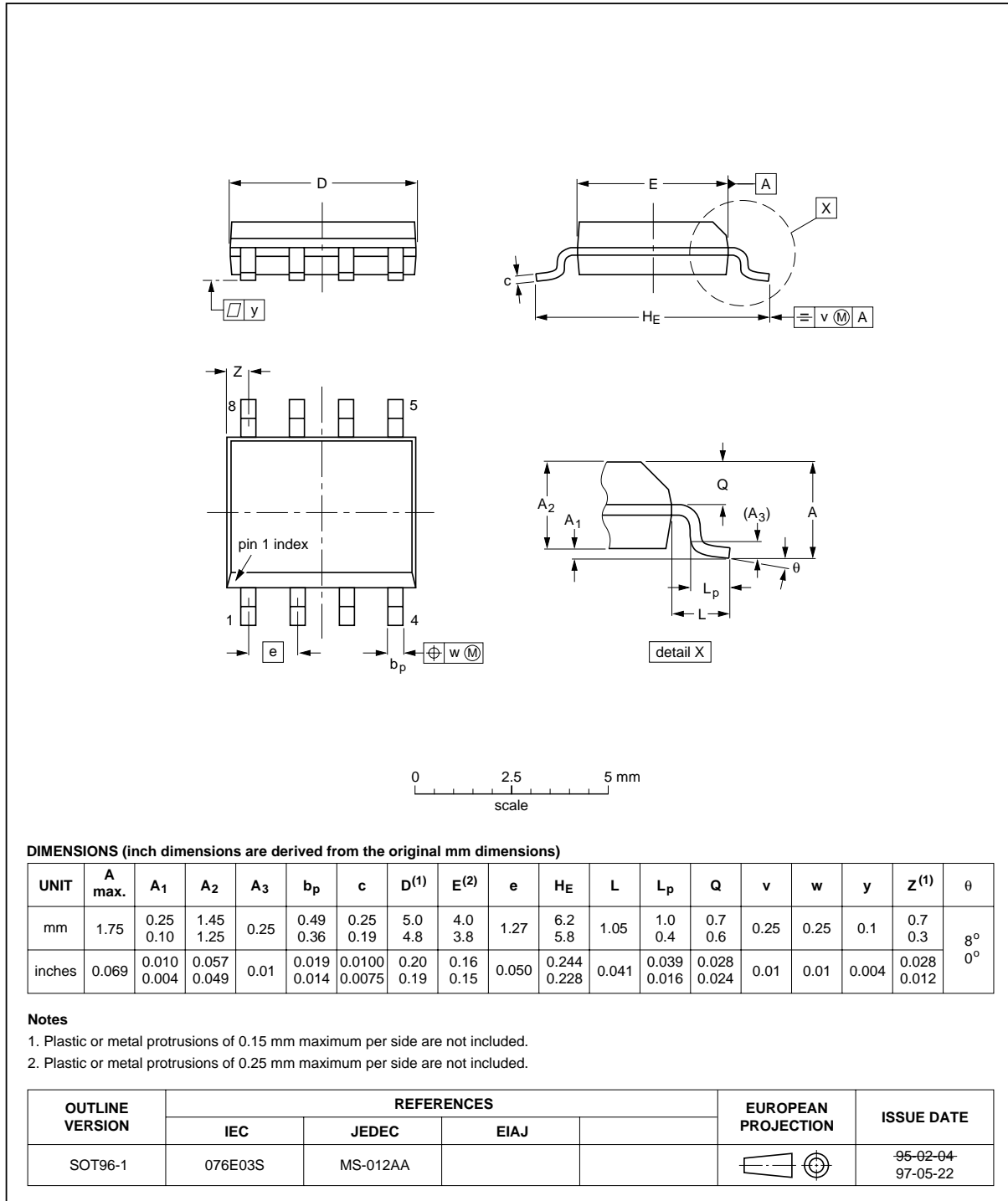
Fig 14. SOT96-1 (SO8).
