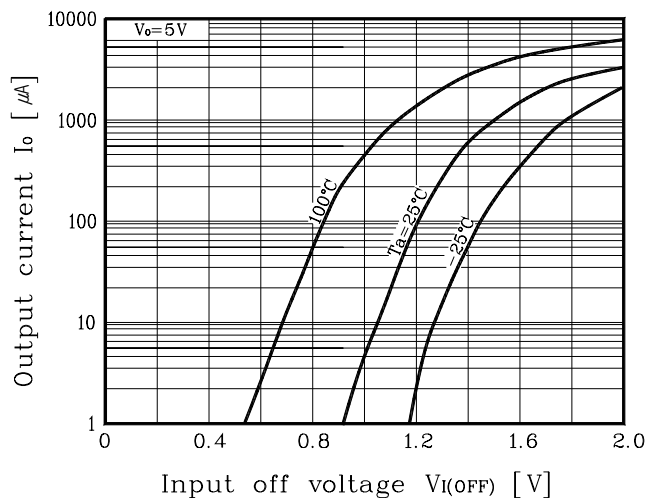
Fig. 3 G_I - I_O
