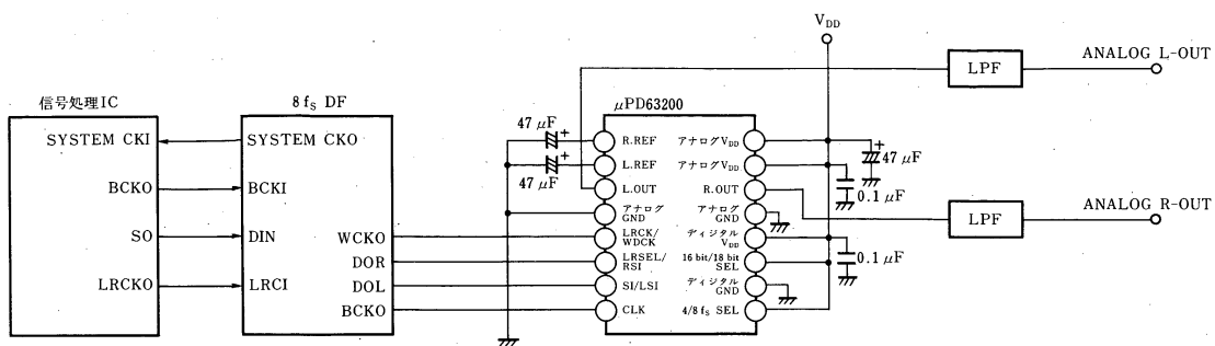
応用回路 (8 f s , 18ビット対応)
