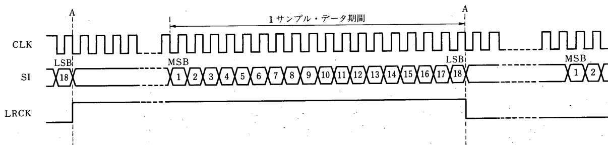
図1 シリアル・データ入力の場合のタイミング・チャート
