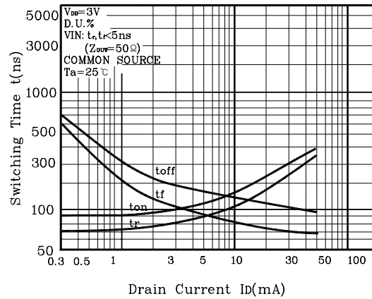
Fig.8 t - I D
