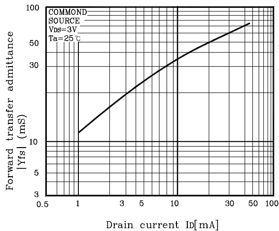
Fig.5 |Y_{fs}| - I_D
