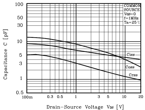
Fig.6 C - V_{DS}
