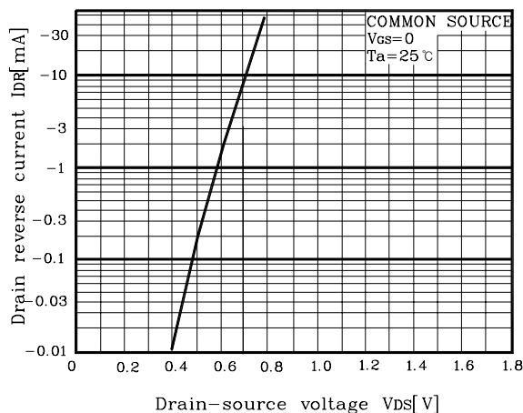
Fig3 I DR - V DS
