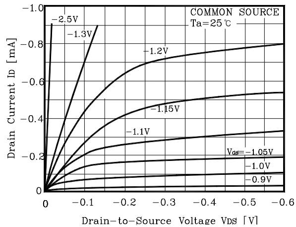
Fig2 I D - V DS
