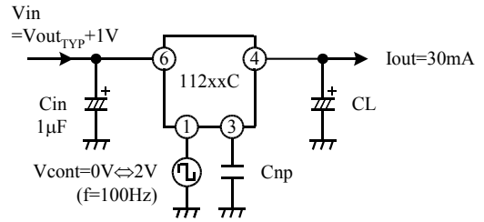
CL=可変 Cnp=0.01 µF
