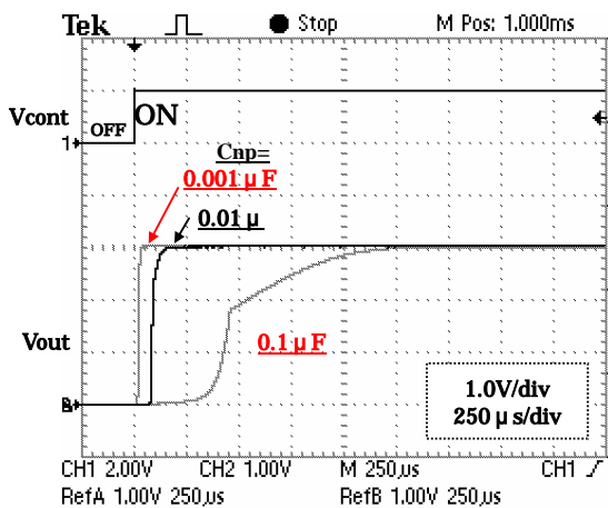
Cnp= 可変 CL=1 µF
