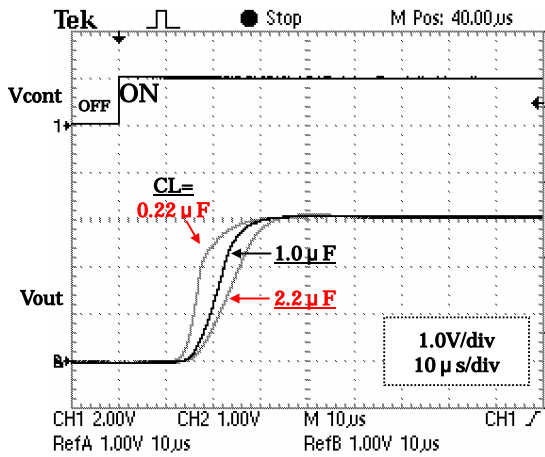
CL= 可変 Cnp=0.001 µF
