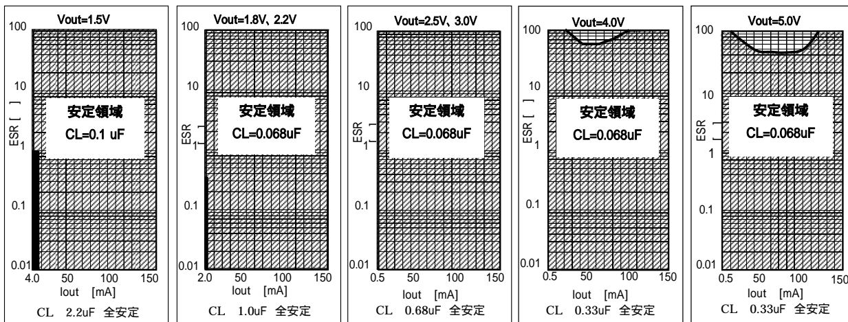
出力電圧、電流 安定動作領域特性
