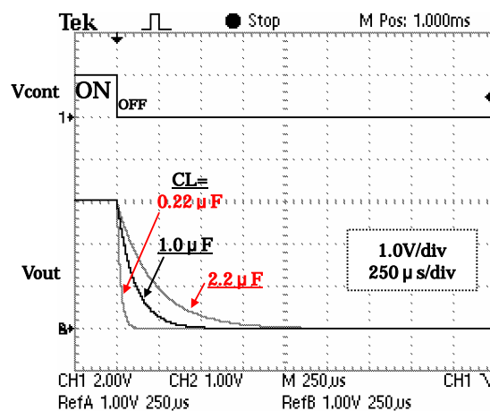
CL= 可変 Cnp=0.01 µF Io=30mA
