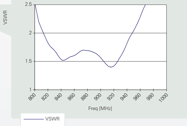
VSWR
