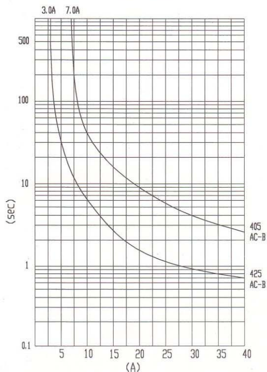
特性曲線圖
