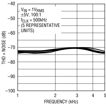
LTC1164-5 • G21
