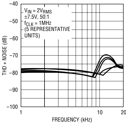
LTC1164-5 • G18
