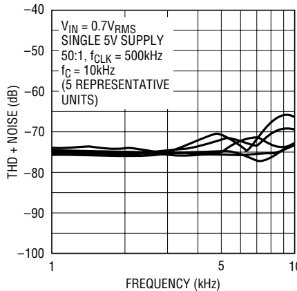
LTC1164-5 • G22
