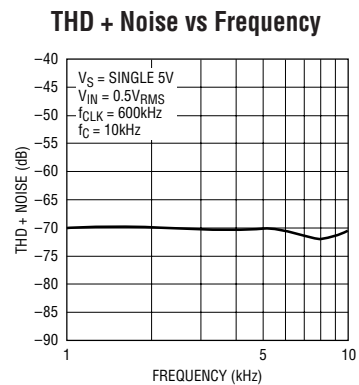
LTC1164-5 • TA04
