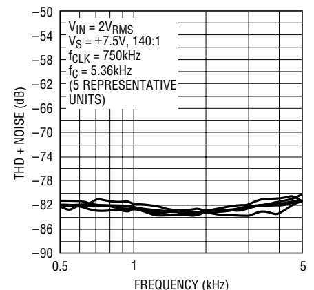
LTC1164-5 • G23
