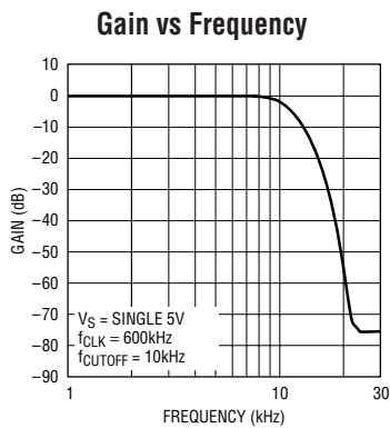
LTC1164-5 • TA03
