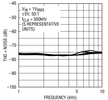
LTC1164-5 • G20
