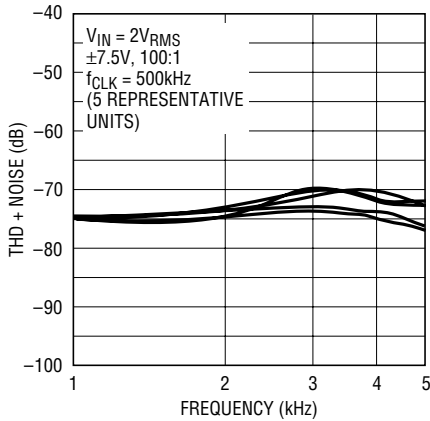
LTC1164-5 • G19
