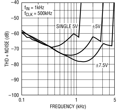
LTC1164-5 • G17
