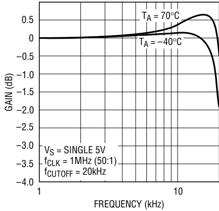
LTC1164-5 • G015
