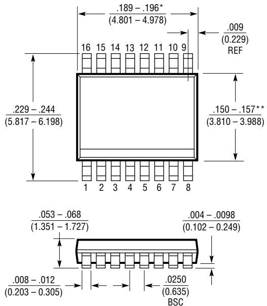
GN16 (SSOP) 0502
