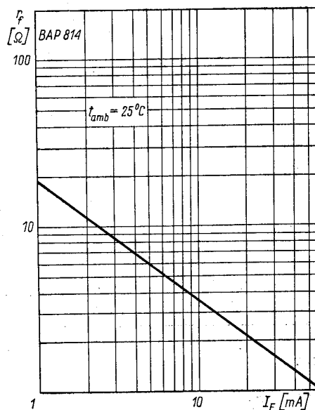
Oporność dynamiczna w funkcji prądu przewodzenia r_f = f(I_F)
