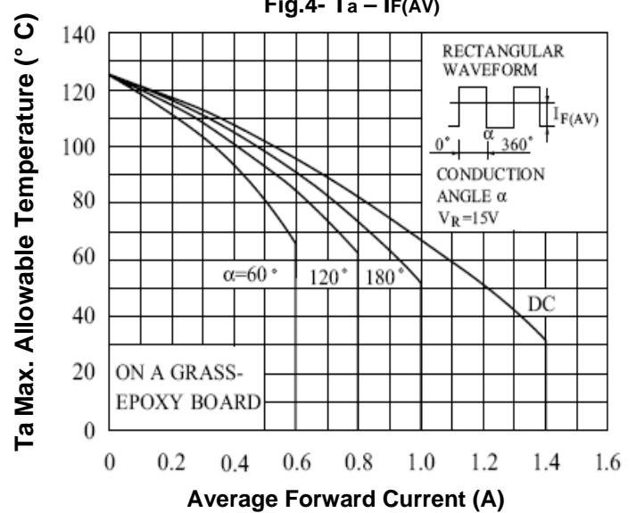
Fig.4- T_a - I_{F(AV)}
