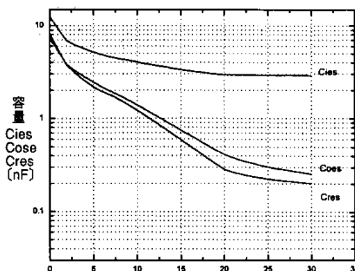
容量-コレクタ・エミッタ間電圧特性 ( T_j=25^{\circ}C ) <INV部> Capacitance vs. Collector-Emitter voltage <INV>
