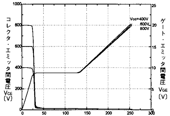
充電電荷量 Q_g(\text{nC}) ダイナミック入力特性 ( T_j=25^\circ\text{C} ) <ブレーキ部> Dynamic input characteristic <BRAKE>
