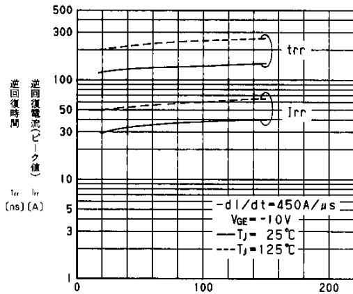
T_{rr} , I_{rr} - I_f 特性 T_{rr} , I_{rr} - I_f
