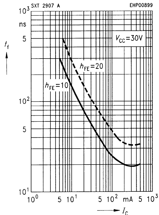
Fall time t_f = f(I_C)
