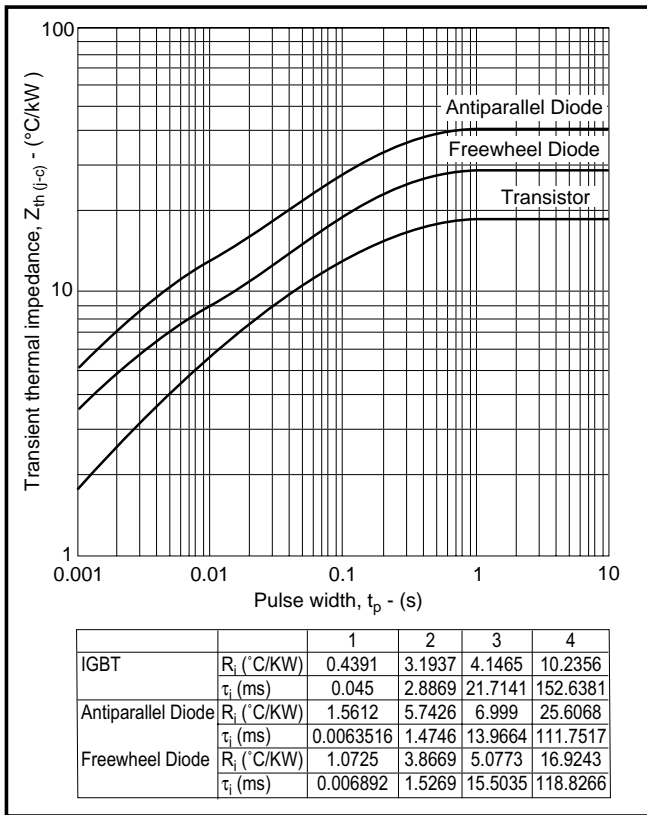
Fig. 13 Transient thermal impedance
