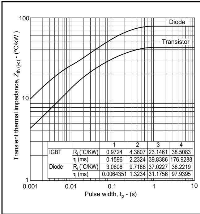
Fig. 13 Transient thermal impedance
