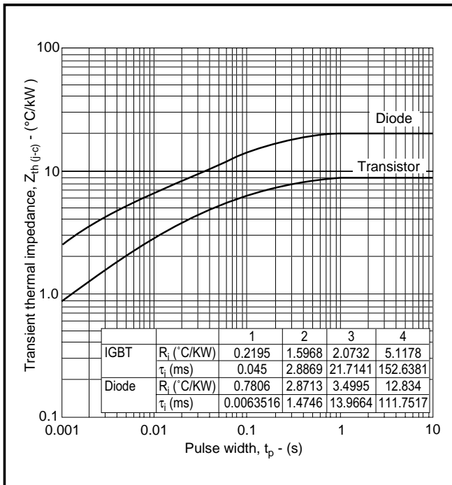
Fig. 11 Transient thermal impedance
