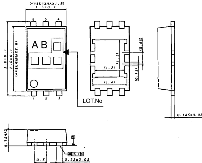
HVSO6 (Unit:mm)
