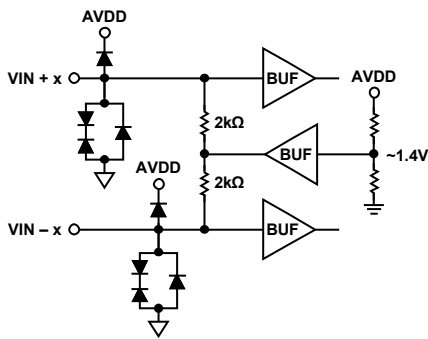
Figure 27. Analog Inputs
