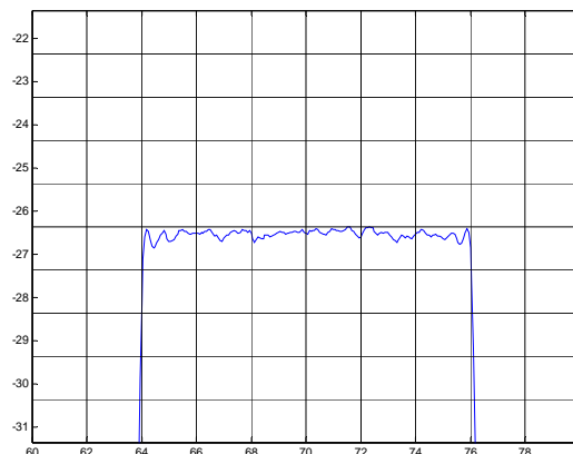
Phase Linearity( f_0 \pm 15\text{MHz} )
