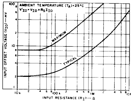
Fig. 16 - Offset error.
