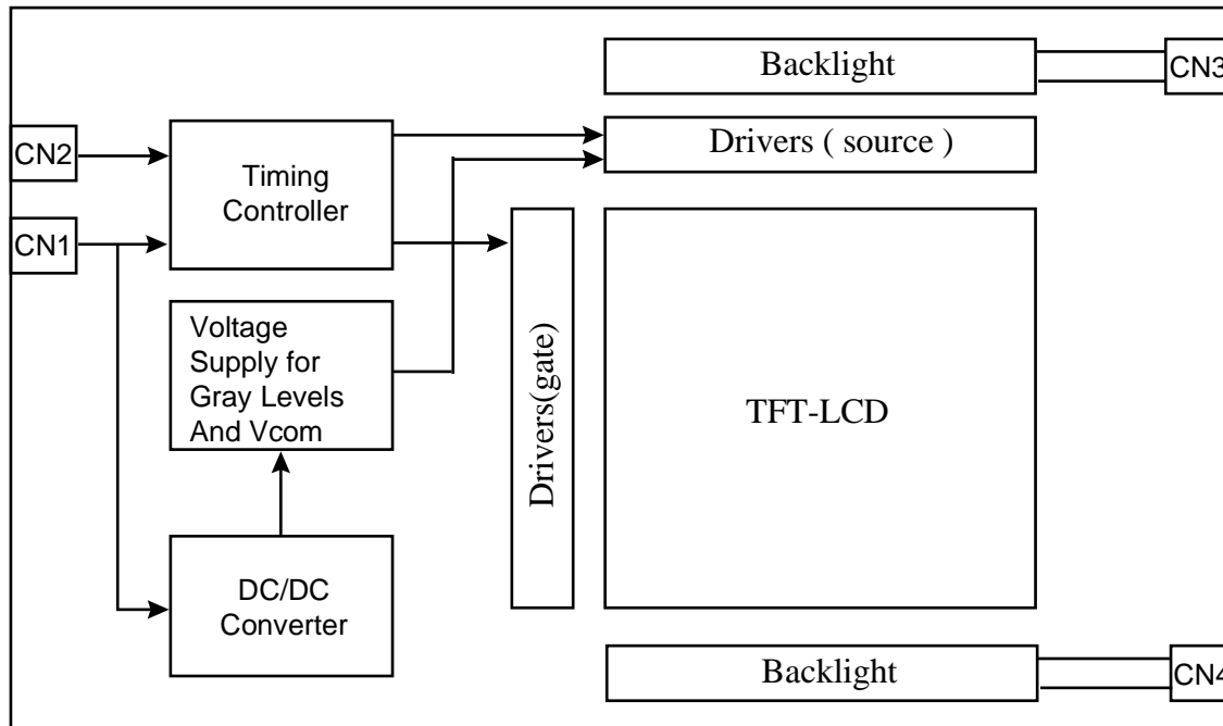
TFT-LCD Module
