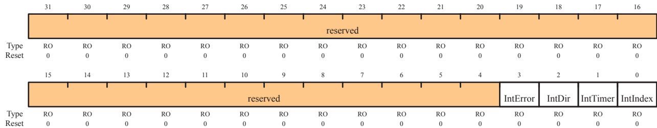
QEI Raw Interrupt Status (QEIRIS)
