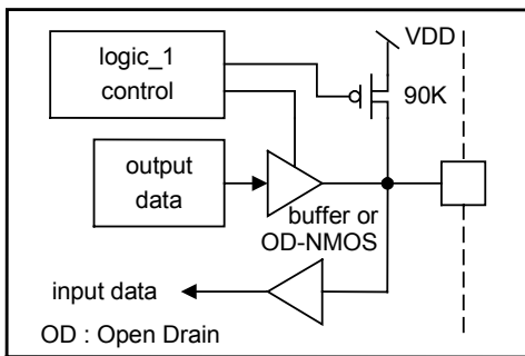
Input/Output IOA port : IOA3 - 0
