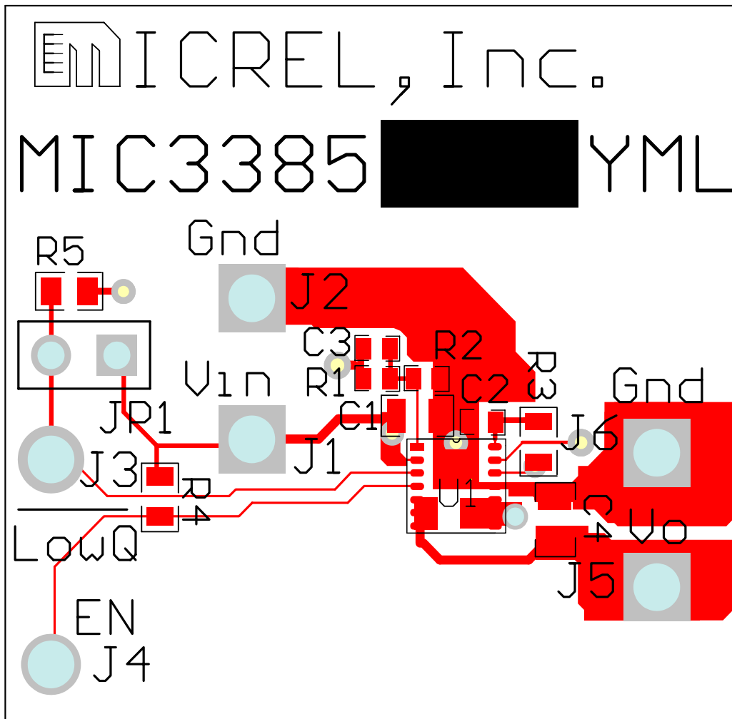
Top Layer
