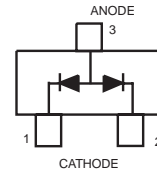
CASE 419-04, STYLE 4 SOT-323 / SC - 70
