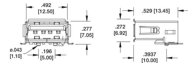
USB-A-S-RA-TSMT
