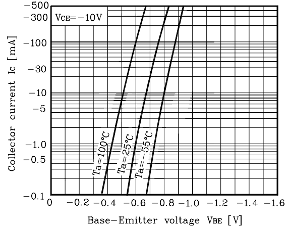
Fig. 2 I_C - V_{BE}
