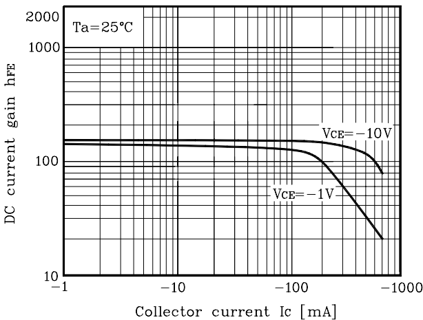
Fig. 5 h_{FE} - I_C
