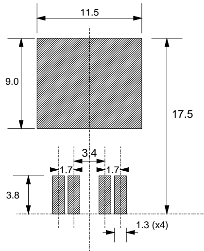
Fig.39. SOT426
