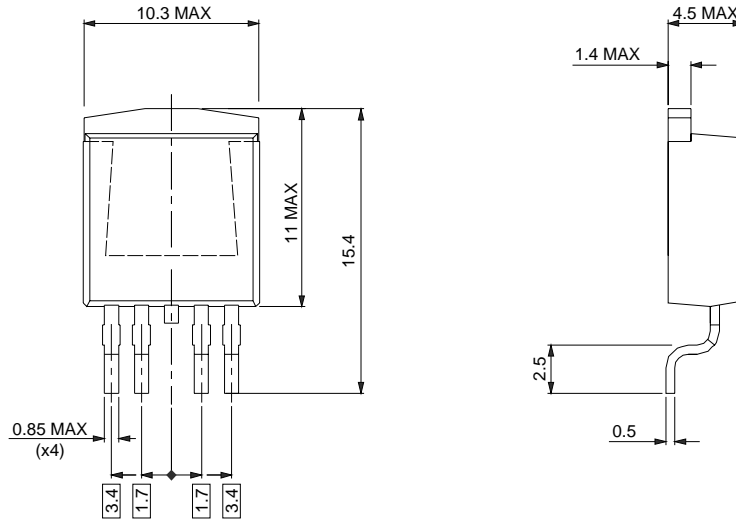
Fig.33. SOT426
