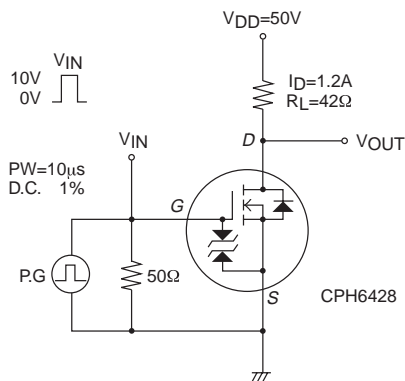
スイッチングタイム測定回路図
