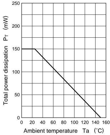
P_T - T_a
