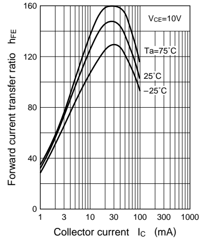
h_{FE} - I_C
