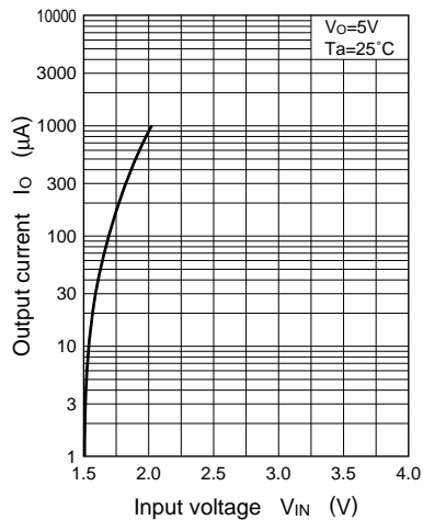
I_O - V_{IN}
