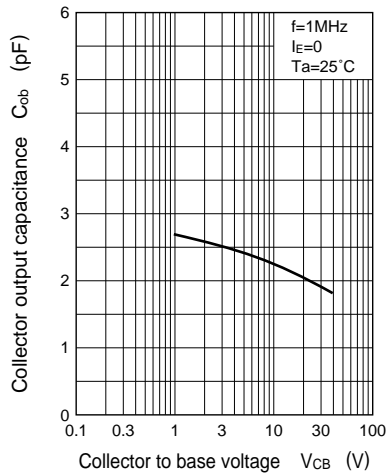
C_{ob} - V_{CB}
