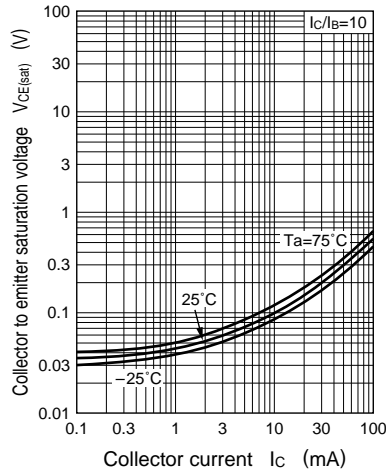
V_{CE(sat)} - I_C
