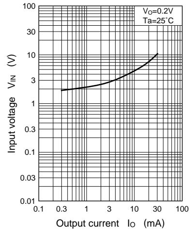
V_{IN} - I_O
