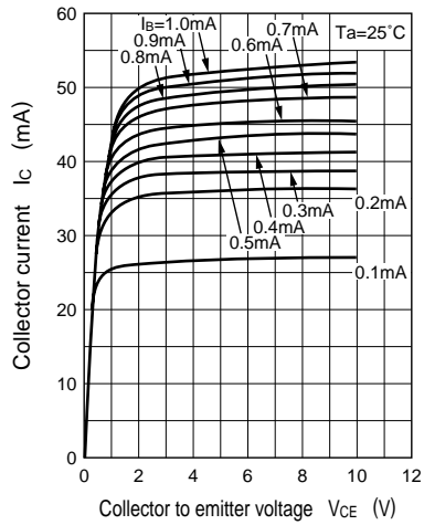
I_C - V_{CE}
