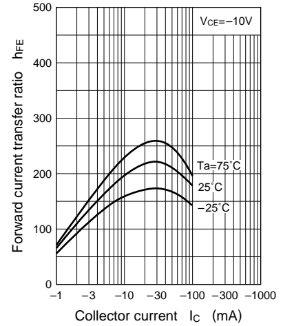
h_{FE} - I_C
