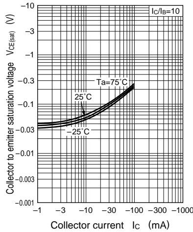
V_{CE(sat)} - I_C
