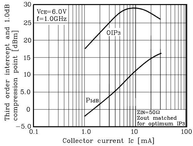
Fig. 18 OIP_3, P_{1dB} - I_C
