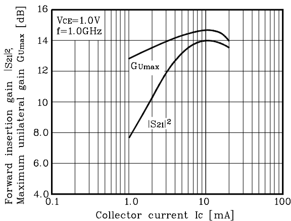
Fig. 10 |S 21 | 2 ,G Umax -I C
