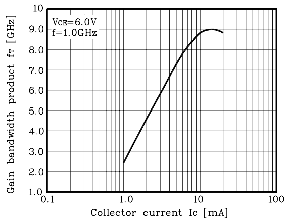
Fig. 4 f_T - I_C
