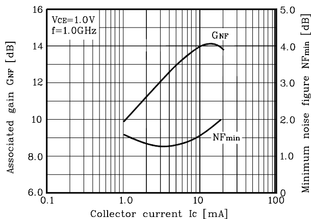
Fig. 16 NF min ,G NF -I c
