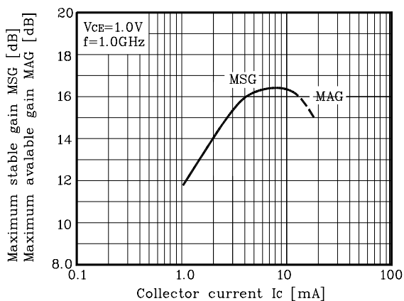
Fig. 12 MSG,MAG-I c
