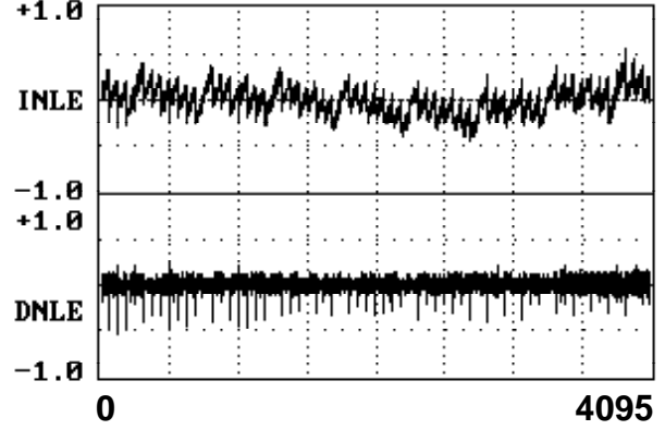
Vcc = 3.30V
