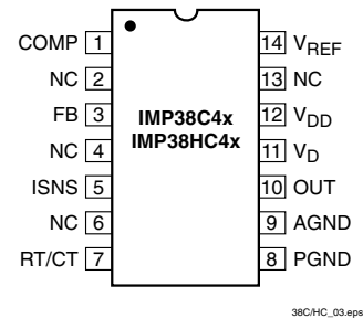
SO/DIP
