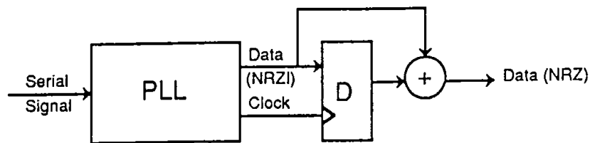
Fig. 9-8. NRZI to NRZ conversion
