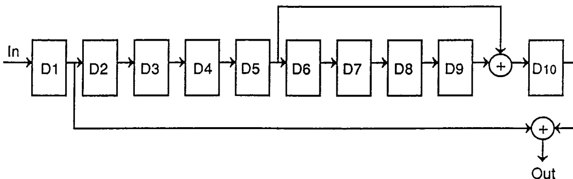
Fig. 9-9 (b). Actual X^9 + X^4 + 1 descrambler
