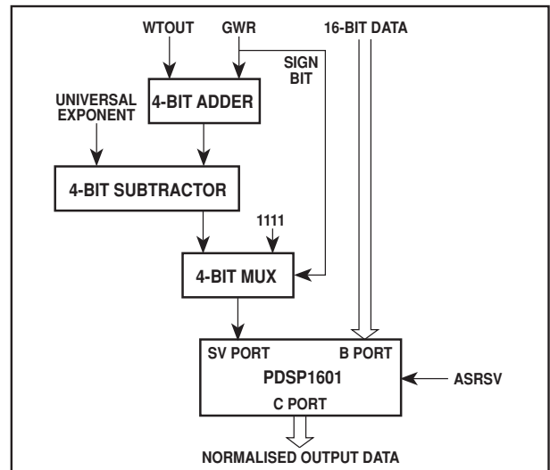
Fig. 8 Output normalisation circuit
