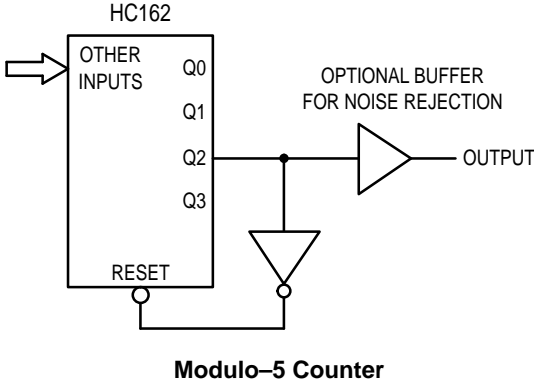
Modulo-5 Counter
