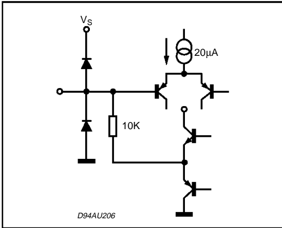
PIN: LP
