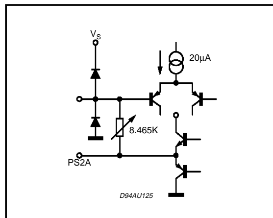
PIN: PS2
