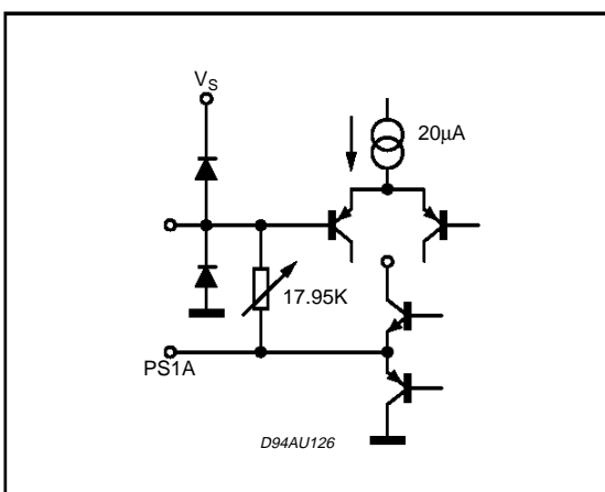
PIN: PS1
