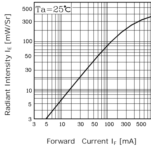
Fig. 2 I_E - I_F
