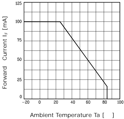
Fig. 3 I_F - T_a
